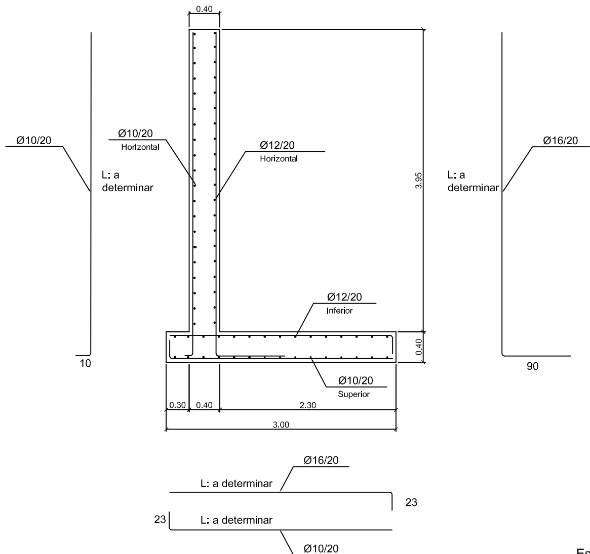
CORTE A-A
