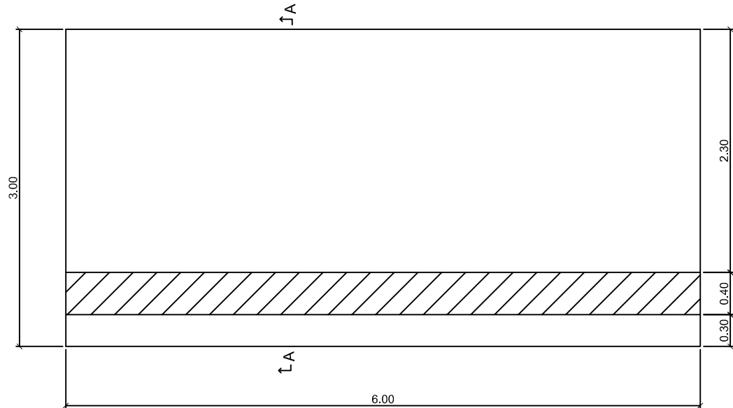
PLANTA
